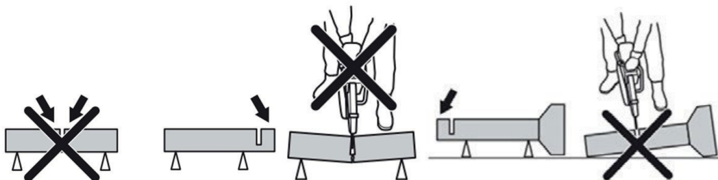
Рис. 21. Блокировка режущего диска
